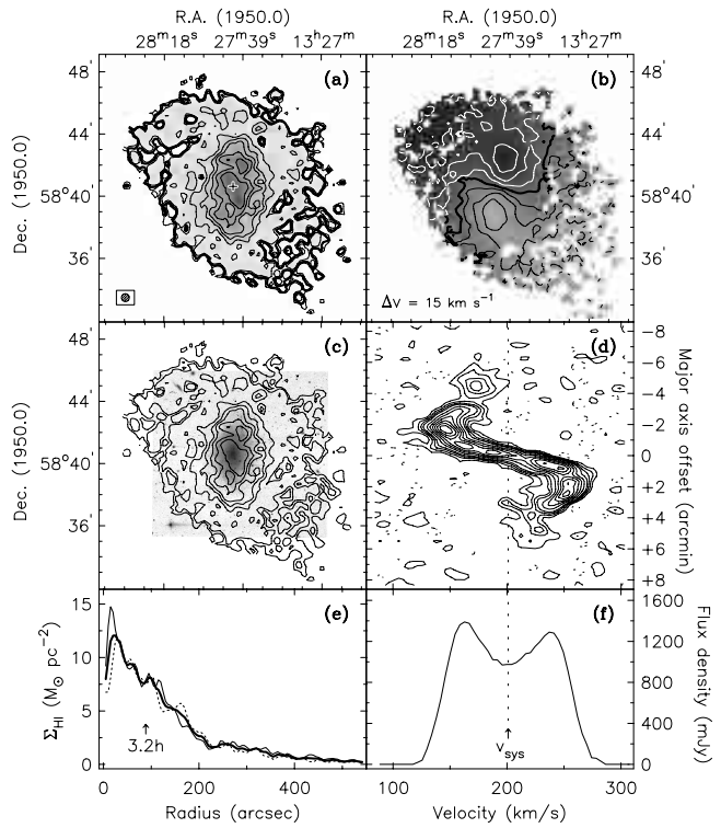
UGC 8490 (NGC 5204)
