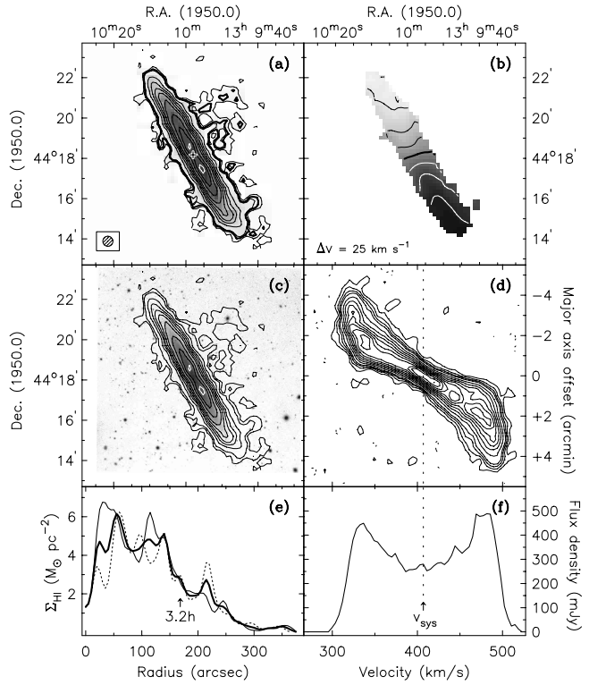
UGC 8286 (NGC 5023)
