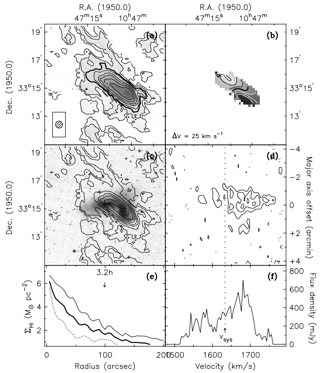
UGC 5935 (NGC 3396)
