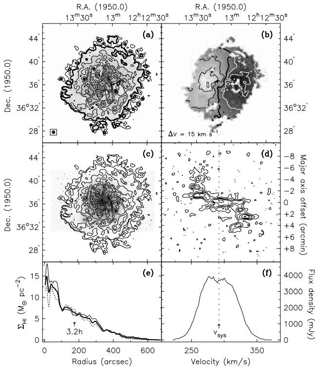
UGC 7278 (NGC 4214)
