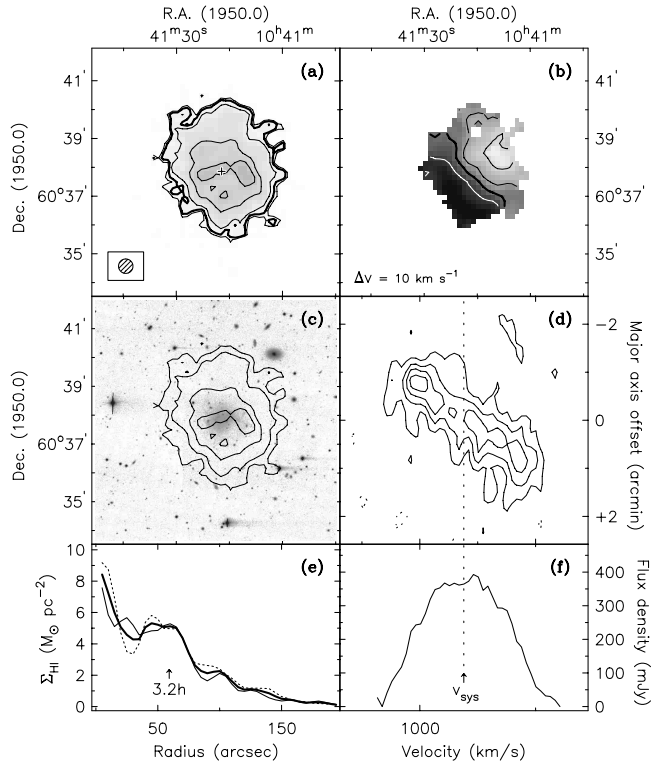
UGC 5846 (DDO 86)
