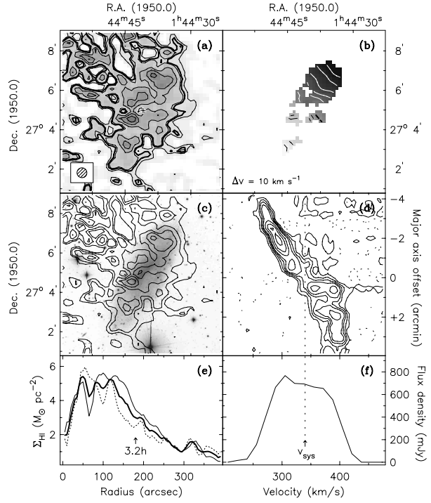
UGC 2023 (DDO 25)
