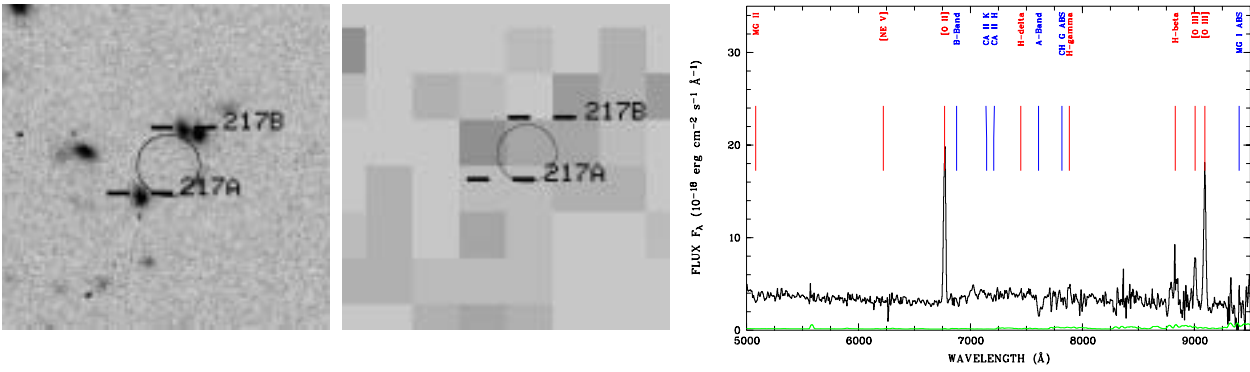
object 217A, z = 0.816
