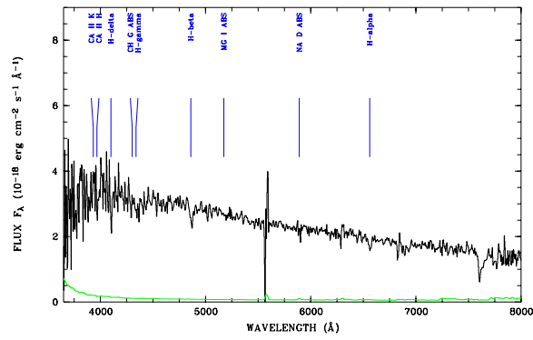
object 3MA, z = 0.000
